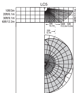
LC5 180° cubierta de lente media luna para HBS 300 (347-480V)
