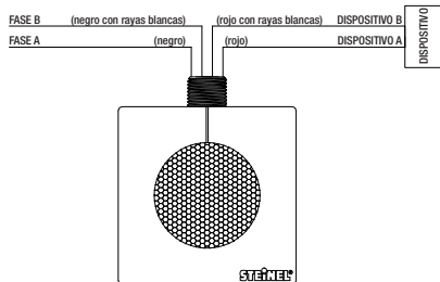
Cableado 347 VCA, 60 Hz
