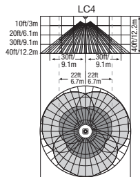
Couvercle de lentille à portée réduite LC4 pour HBS 300 (347-480V)
