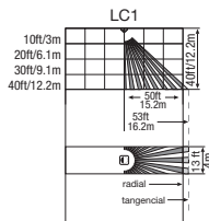
LC1 cubierta inicial de pasillo para HBS 200 (347-480V)
