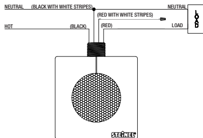
347 VAC, 60 Hz Wiring
