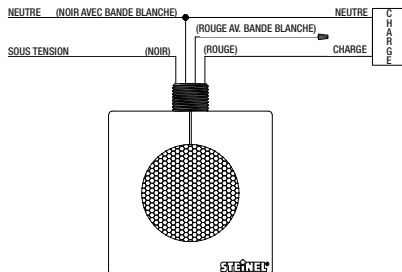
Conducteur 347 VCA, 60 Hz
