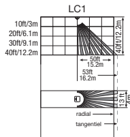
Couvercle de début de couloir LC1 pour HBS 200 (347-480V)
