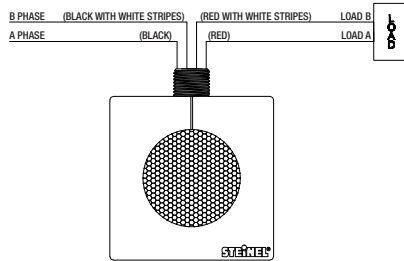
347 VAC, 60 Hz Wiring
