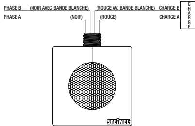
Conducteur 347 VCA, 60 Hz
