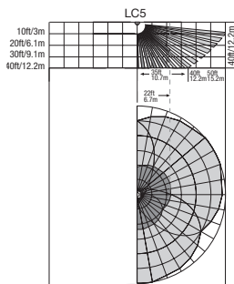
Couvercle de lentille en demi-lune 180° LC5 pour HBS 300 (347-480V)
