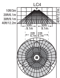
LC4 cubierta de lente con campo reducido para HBS 300 (347-480V)
