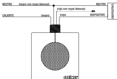
Cableado 347 VCA, 60 Hz
